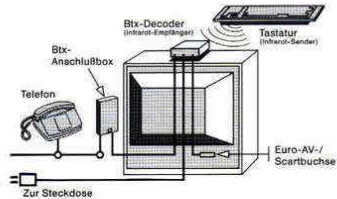
Anschlußschema für das Btx-TV-Set
